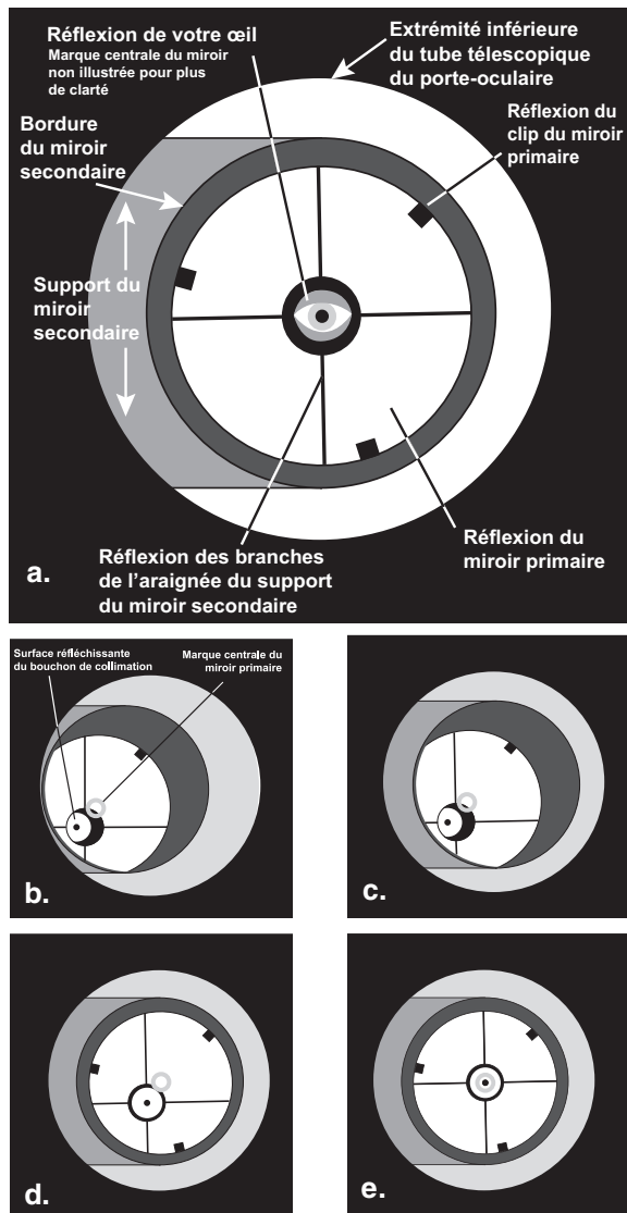
Figure 8. Collimation de l'optique. (a) Lorsque les miroirs sont correctement alignés et que vous regardez à travers le tube télescopique du porte-oculaire, vous devriez voir quelque chose comme ceci. (b) L'ocillet de collimation étant en place, la vue peut ressembler à ceci, si l'optique est désalignée. (c) Ici, le miroir secondaire est centré sous le porte-oculaire, mais il doit être ajusté (incliné) de manière à ce que le miroir primaire soit visible dans sa totalité. (d) Le miroir secondaire est correctement aligné, mais le miroir primaire doit toujours être ajusté. Lorsque le miroir primaire est correctement aligné, le « point » est centré, comme illustré en (e).
