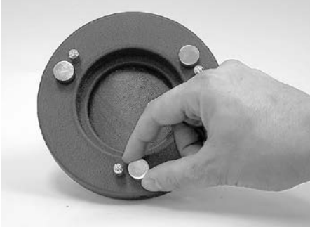
Figure 12. L'inclinaison du miroir primaire est ajustée en tournant une ou plusieurs des trois grosses vis de collimation.
