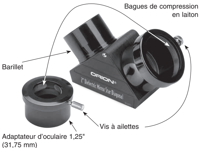
Le diagonal à miroir haute réflectivité 2" (50,80 mm) d'Orion
