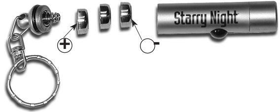
Figure 1. Le pôle positif (+) de l'ensemble des trois piles doit être du côté de la chaînette au bout de la mini-torche et le pôle négatif (-) de la batterie du côté de la LED, à l'avant de la mini-torche.
