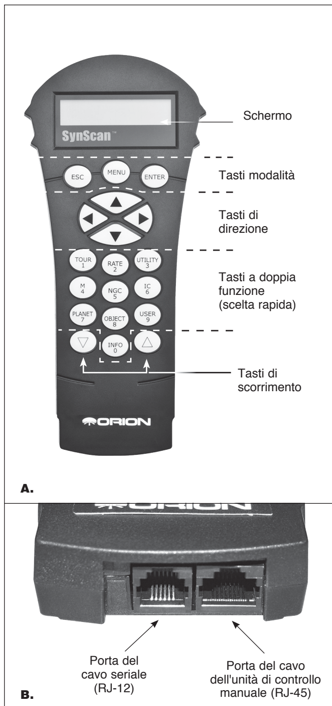
Figura 17. A) Unità di controllo manuale GoTo SynScan, B) Porte dei cavi seriale e dell'unità di controllo manuale sull'estremità inferiore dell'unità di controllo.
