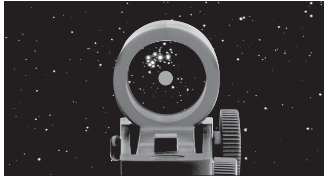
Figura 12. Inserire il mirino EZ Finder II nel supporto a coda di rondine orientandolo come indicato e fissarlo con la vite zigrinata.
