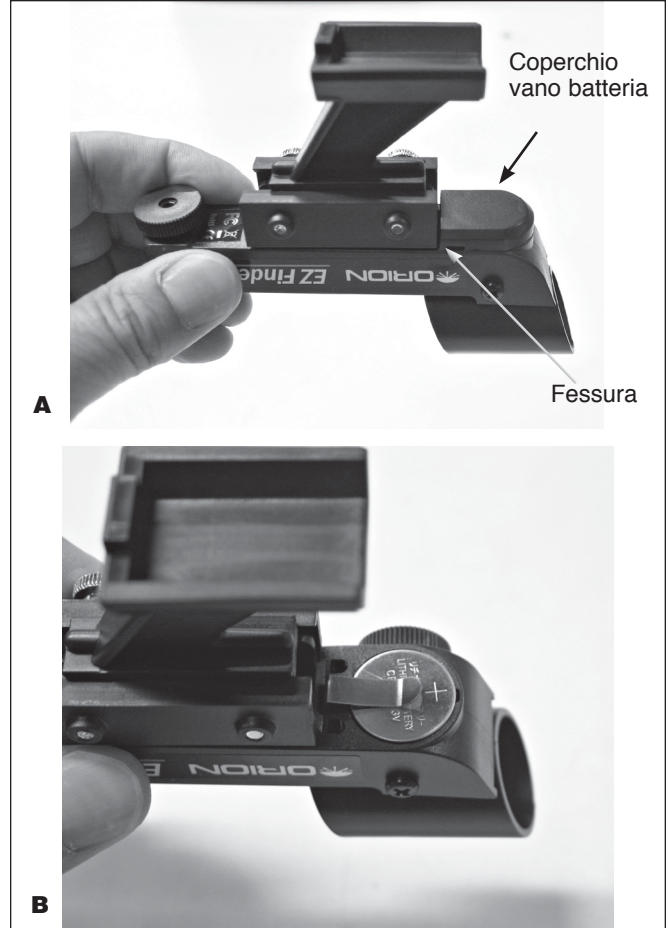
Figura 10. A) Per installare la batteria CR2032 del mirino EZ Finder II, girarlo a testa in giù e rimuovere il coperchio del vano batteria. B) Installare la batteria con il lato positivo (+) rivolto verso l'alto, come mostrato.
