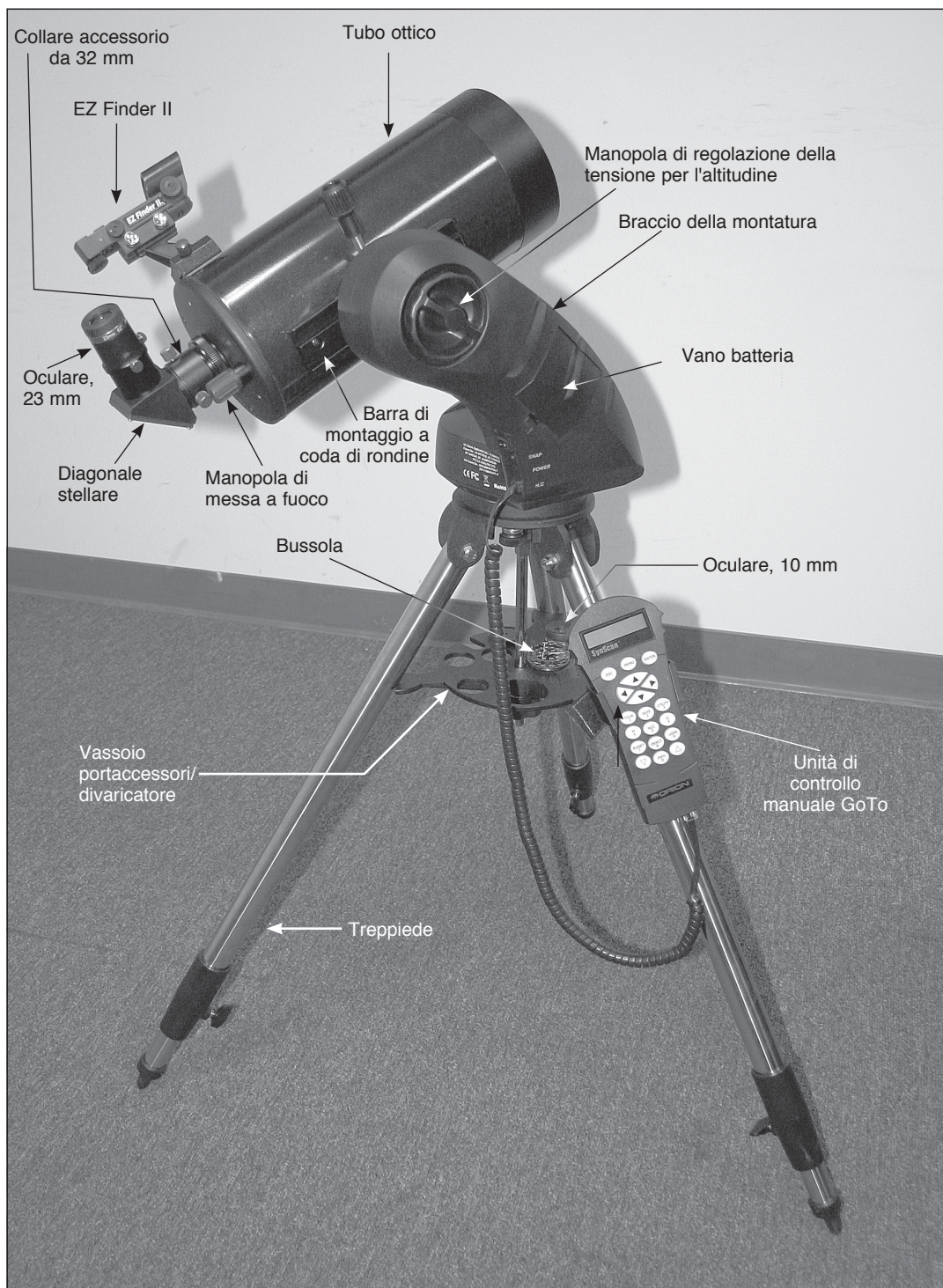
Figura 1. Componenti dello StarSeeker IV (in figura Maksutov-Cassegrain 127 mm)
