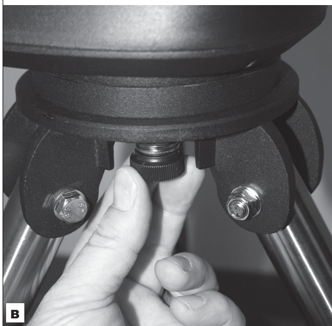
Figura 4. Il braccio della montatura si fissa alla piattaforma di montaggio del treppiede con tre bulloni imperdibili. A) Allineare i bulloni ai fori nella parte inferiore della base del braccio. B) Serrare le tre manopole.
