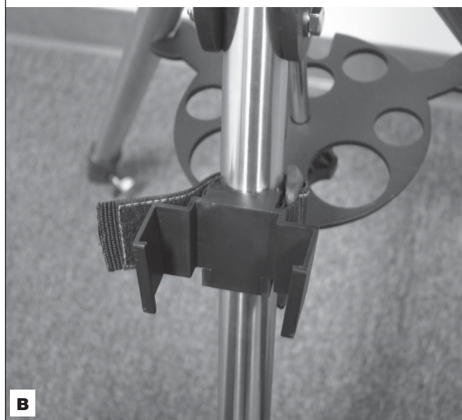
Figura 5. A) Avvolgere la cinghia intorno a una gamba del treppiede e tirare fermamente prima di fissare. B) Supporto dell'unità di controllo manuale installato.
