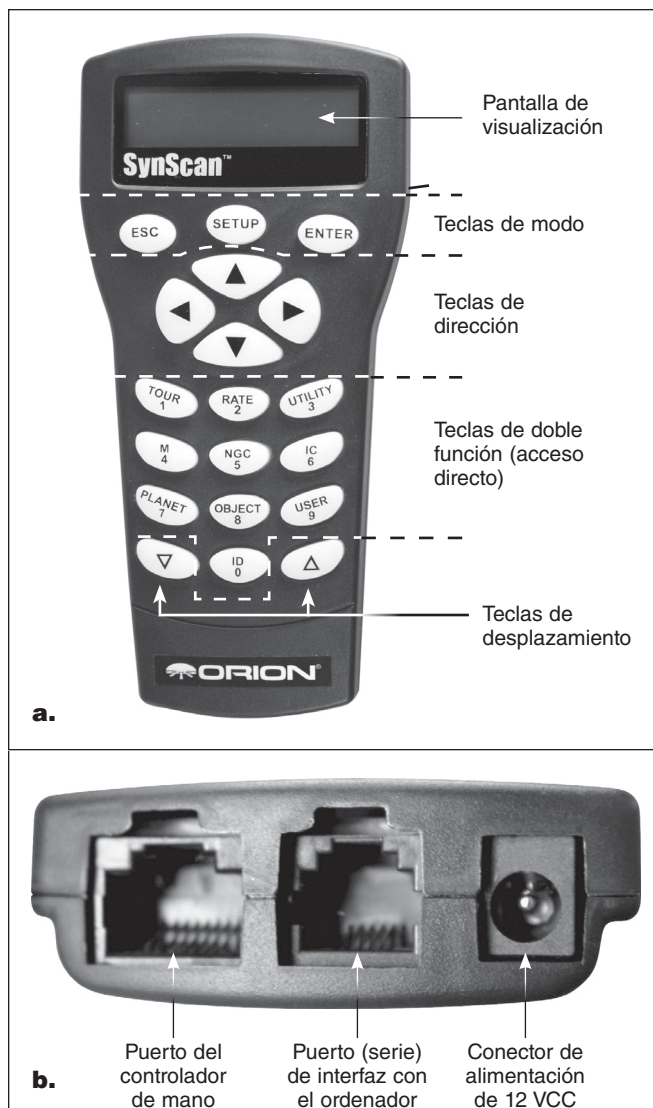
Figura 1. a) Controlador de mano SynScan GoTo. b) Puertos de conexión en la parte inferior del controlador.
