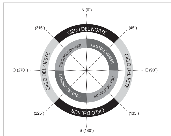
Figura 2. Regiones direccionales del cielo utilizadas en el método de alineación "Estrella más brillante".
