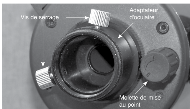
Figure 7. Détail de l'adaptateur d'oculaire du TableTop 90
