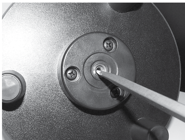
Figure 9b : retrait de l'adaptateur 1/4" -20" (6,4 mm, 20 filets au pouce)
